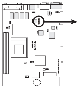
MES-N LCD Header
